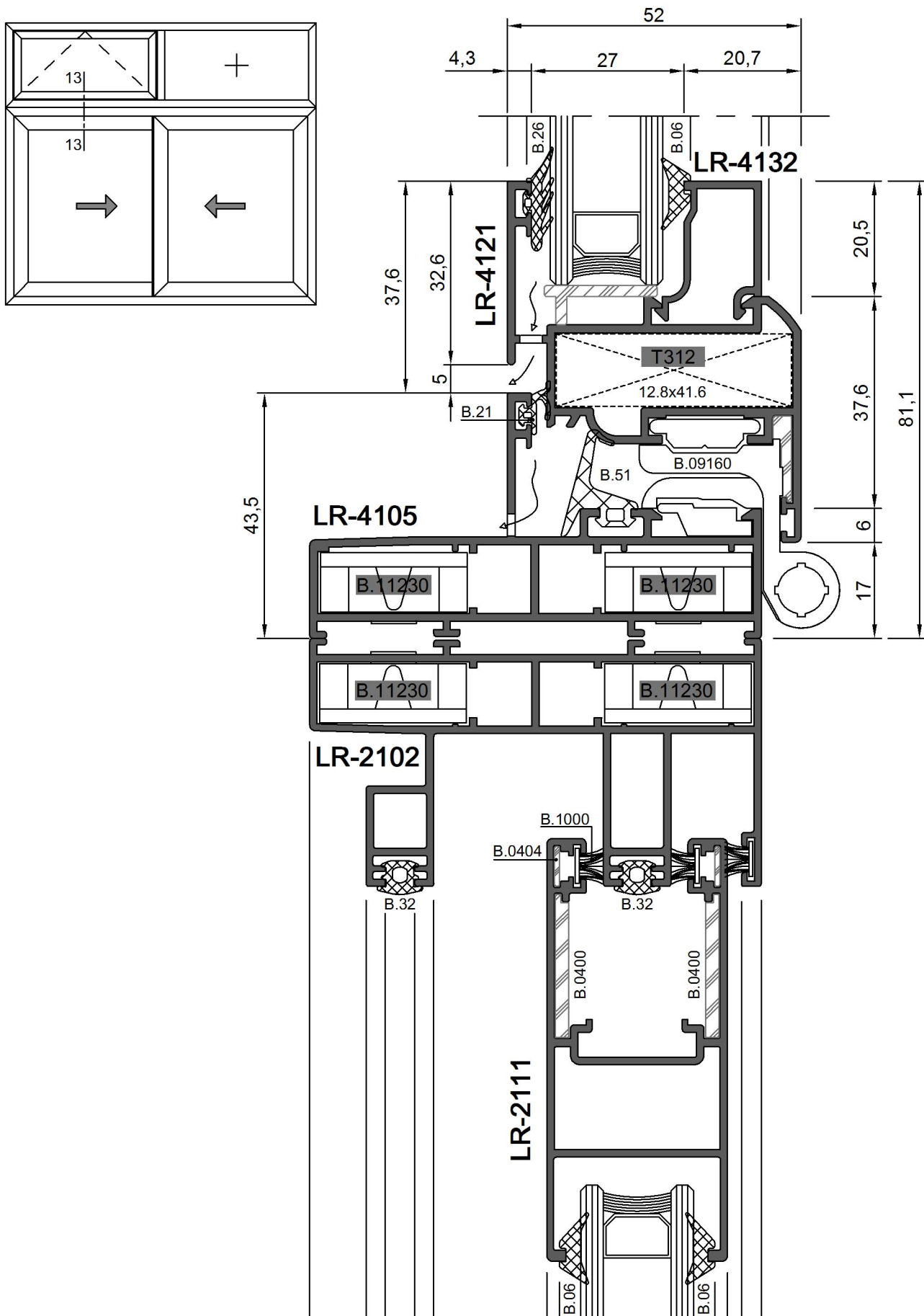
13 - 13 DETAY
