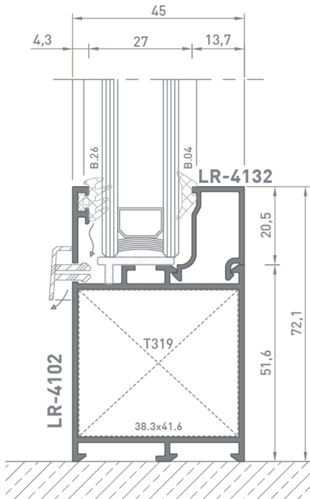
1 - 1 DETAY
