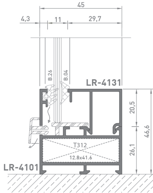
1 - 1 DETAY
