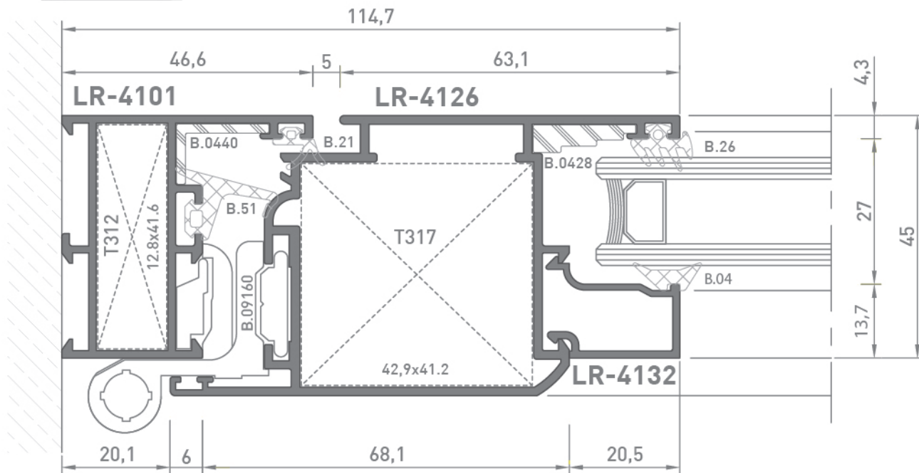
5 - 5 DETAY
