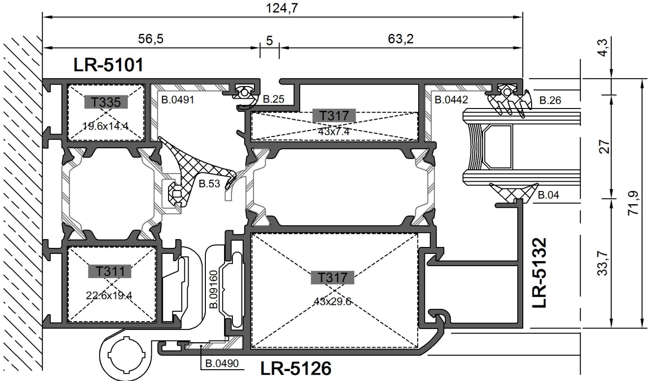
7 - 7 DETAY
