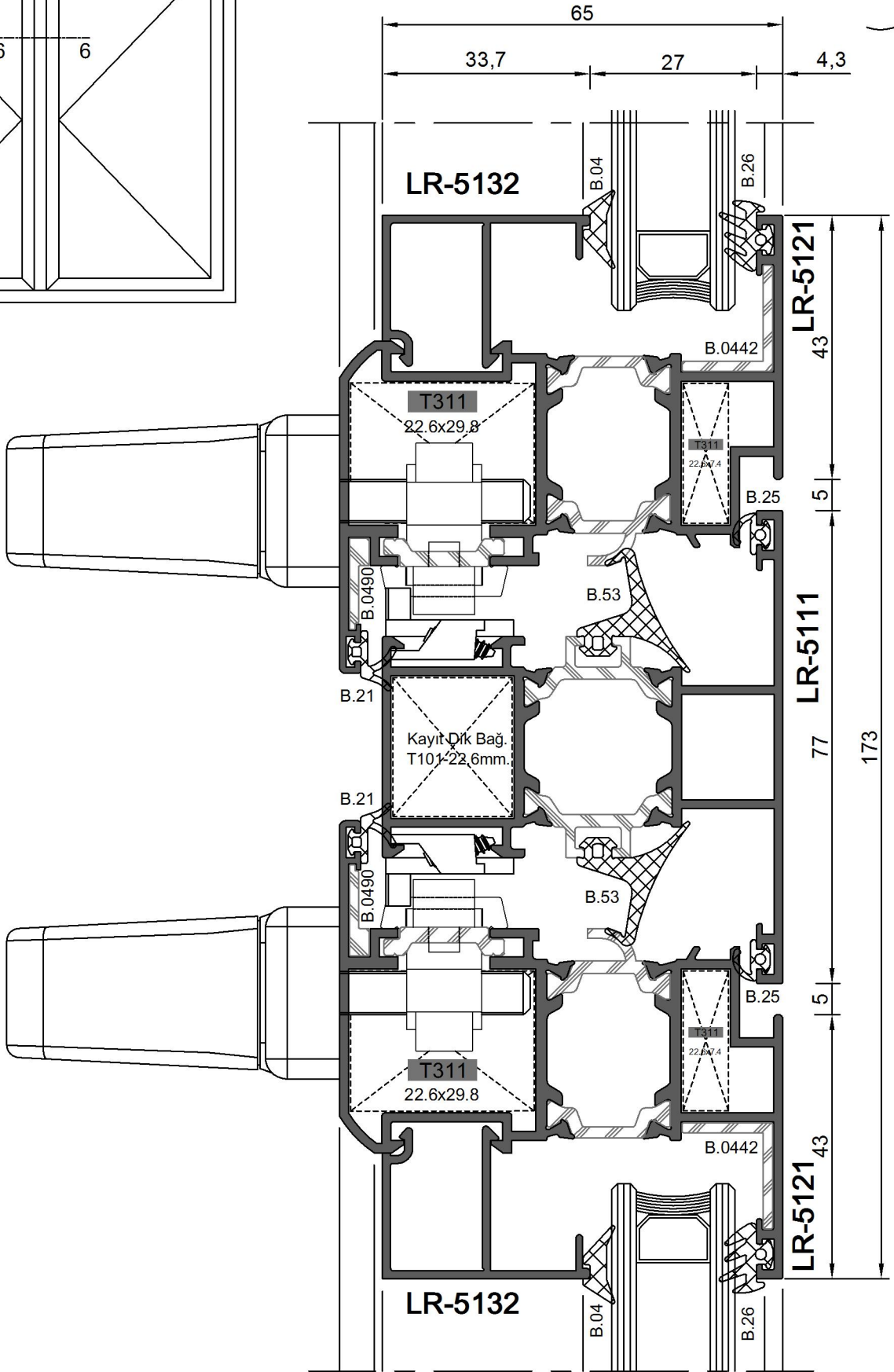
6 - 6 DETAY
